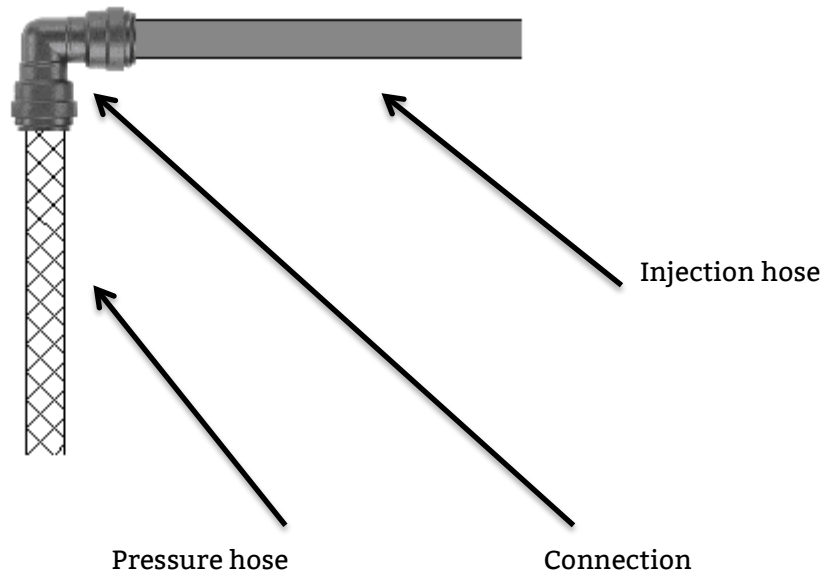
INJECTOTUBE
